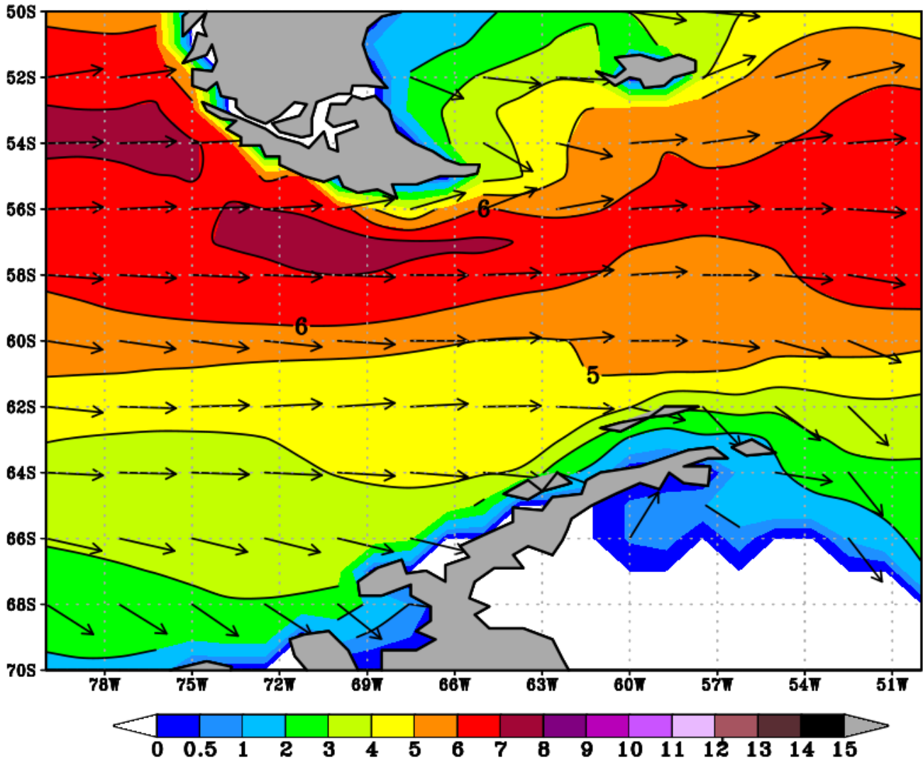
ALTURA DE OLA SIGNIFICATIVA, EN METROS Datos grib Modelo Global NWW3 corrida 06Z10MAR2021 res 0.5°x0.5° procesado con GrADS
